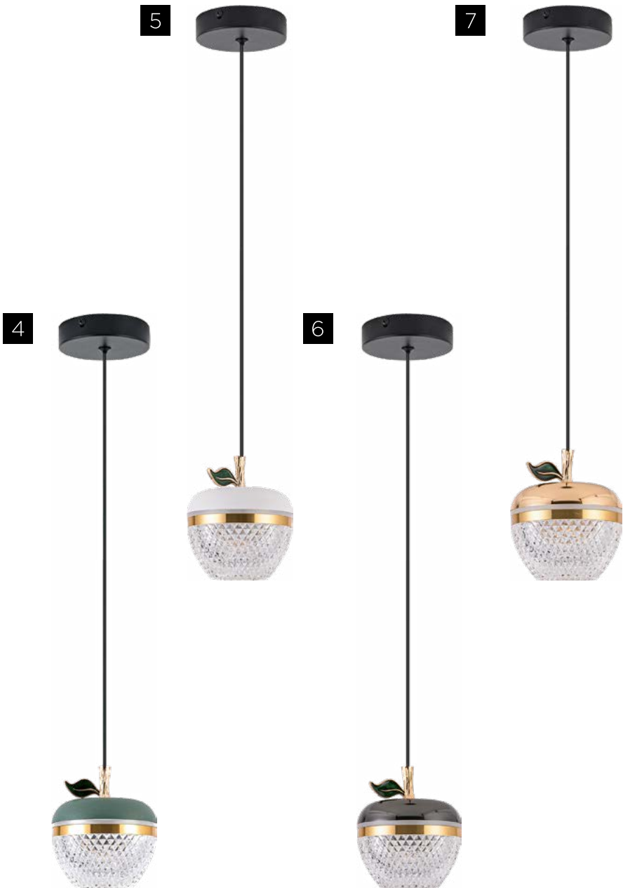
4 L7120-1 GN D100*H1500mm Тип лампы: LED Общая мощность: 7W Цвет. температура: 4000K Цвет: зеленый Материал: металл/акрил
