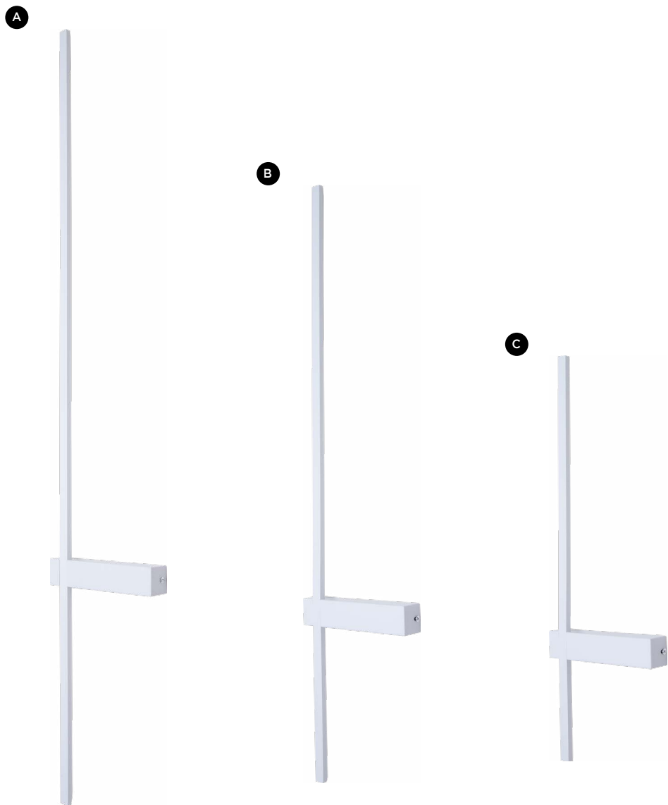
A L7365-1200 WH L200*W35*H1200mm Тип лампы LED Общая мощность 33W Цвет белый Материал металл
