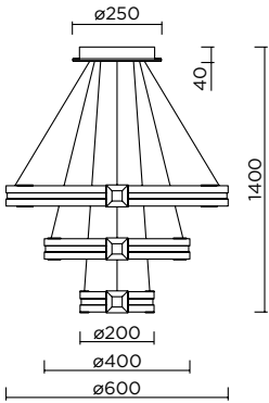
C L77085-3 D600*H300-1400mm Тип лампы LED Цвет. температура 3000-6000K Общая мощность 110W Цвет черный/латунь Материал металл/акрил
