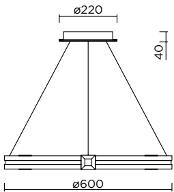
A L77084-1 D600*H300-1400mm Тип лампы LED Цвет. температура 3000-6000K Общая мощность 60W Цвет черный/латунь Материал металл/акрил
