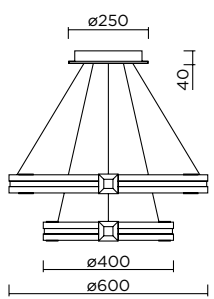
D L77085-2 D600*H300-1400mm Тип лампы LED Цвет. температура 3000-6000K Общая мощность 85W Цвет черный/латунь Материал металл/акрил
