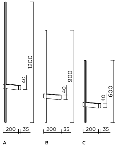
C L7365-1 WH L200*W50*H600mm Тип лампы LED Общая мощность 17W Цвет белый Материал металл
