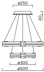
B L77084-2 D520*H300-1400mm Тип лампы LED Цвет. температура 3000-6000K Общая мощность 75W Цвет черный/латунь Материал металл/акрил
