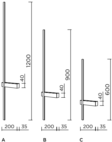
B L7365-900 BK L200*W35*H900mm Тип лампы LED Общая мощность 25W Цвет черный Материал металл
