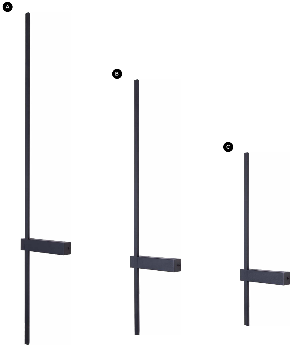
A L7365-1200 BK L200*W35*H1200mm Тип лампы LED Общая мощность 33W Цвет черный Материал металл
